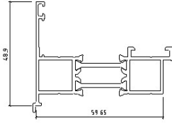
转轴米重: 0.988 KG/M
