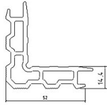
角钢002米重: 1.596 KG/M
