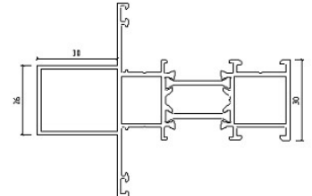
加强中板米重: 1.623 KG/M
