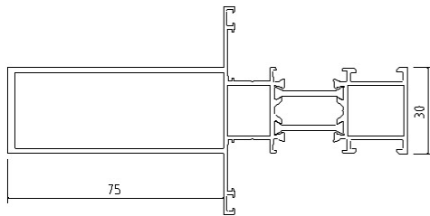
加强中板米重: 2.23 KG/M
