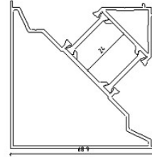
90° 转角/米重: 1.605 KG/M
