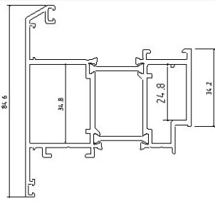
外开门扇/米重: 2.044 KG/M
