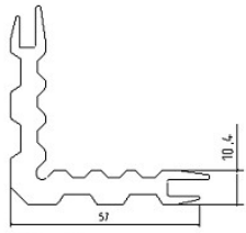
角钢001米重: 2.027 KG/M
