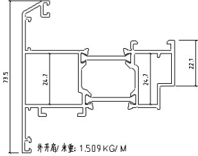
外开扇/米重: 1.509 KG/M
