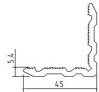
抄扁角钢: 0.845 KG/M
