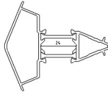
45° 转角/米重: 1.102 KG/M
