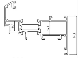
内开扇米重: 1.326 KG/M
