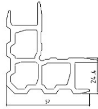
角钢003米重: 2.100 KG/M
