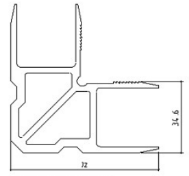
角钢004米重: 2.660 KG/M
