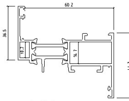
内开扇米重: 1.165 KG/M
